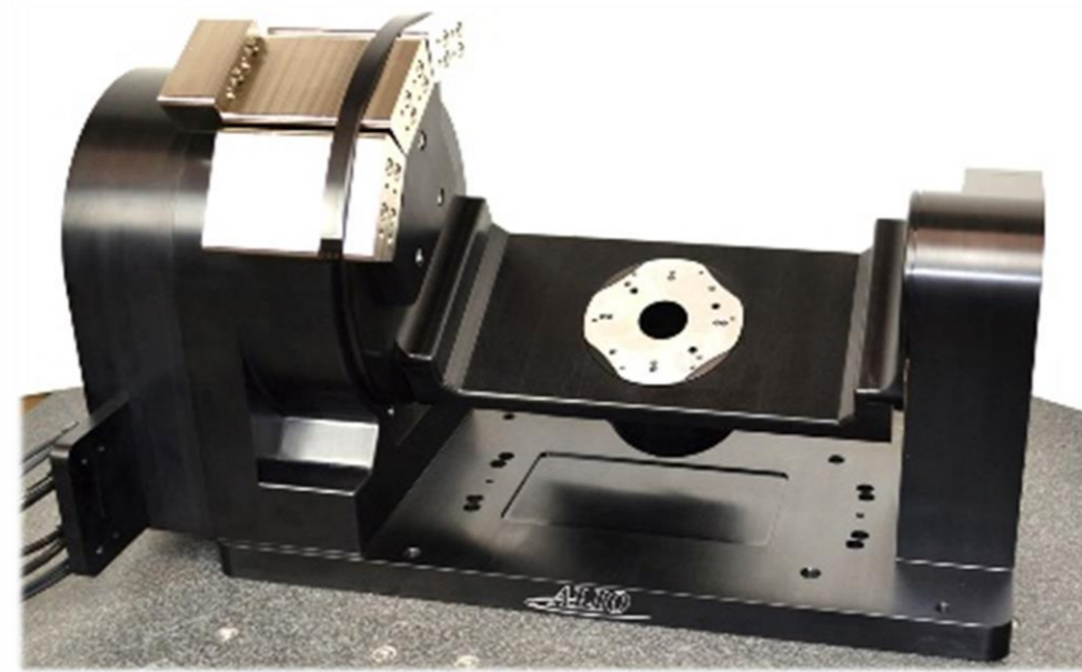
2-Achs kardanische Aufhängung (Gimbal)
