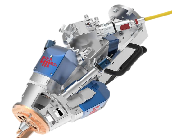
Richtungsunabhängiges Drahtauftragsschweißen bis 30 kW
