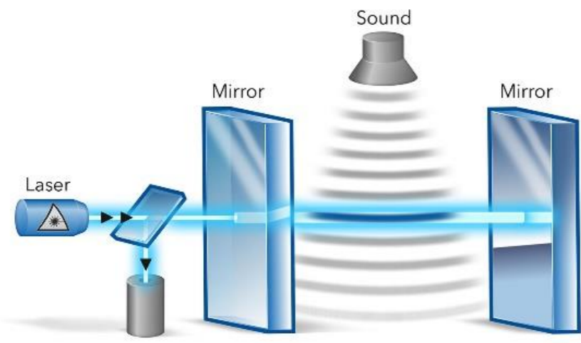
Prinzipdarstellung
